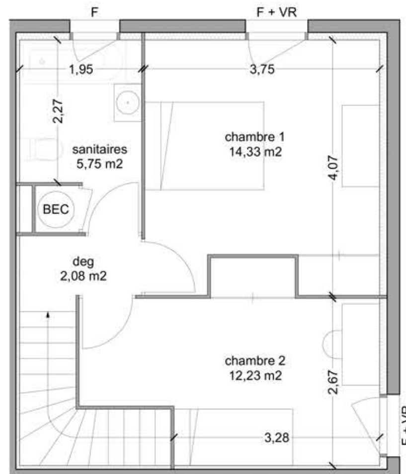
plan étage ech 60e
