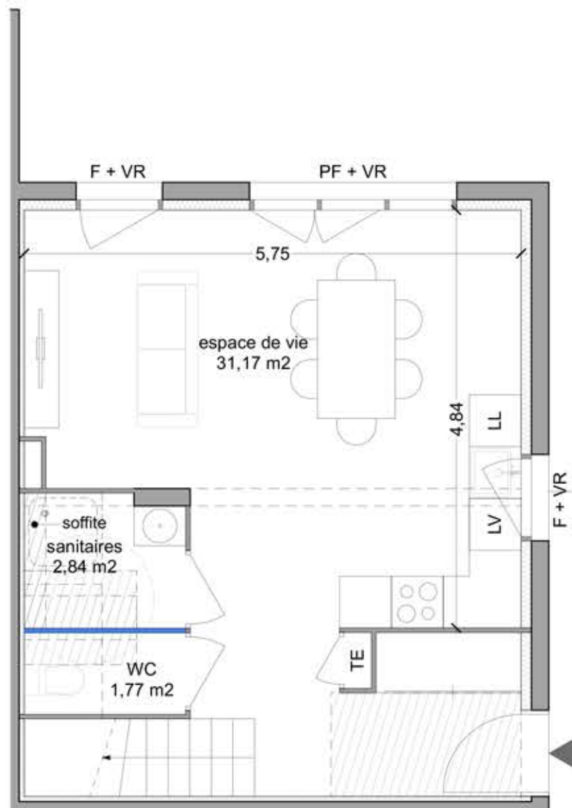
plan RdC ech 60e
